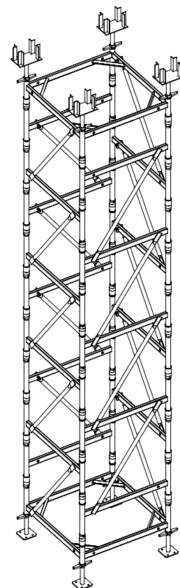
Wieża podporowa S10 - schemat
