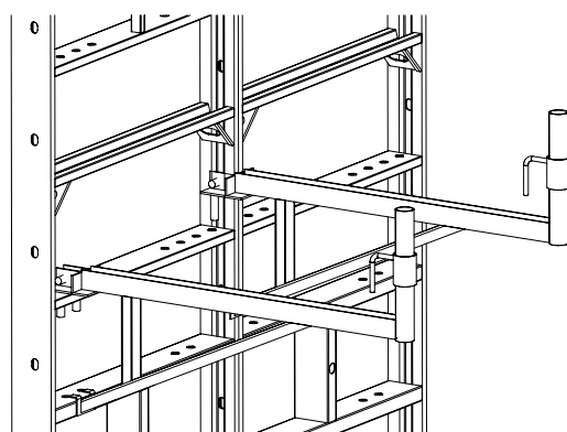
Schemat - montaż pomostów roboczych
