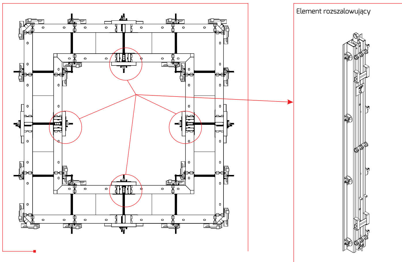
Szalunek szybu windowego - schemat
