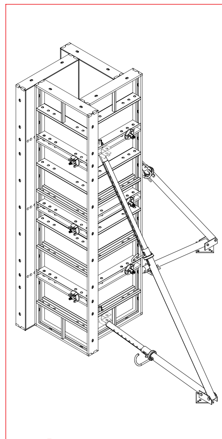
Schemat formowania słupów
