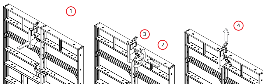
Hak transportowy - zastosowanie
