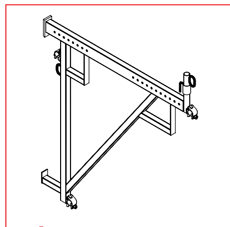
Wspornik szalunku wspinającego
