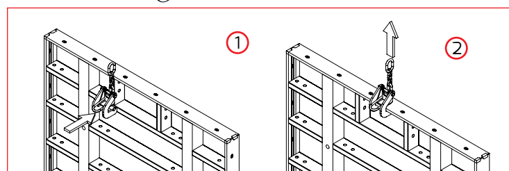
Zawiesie transportowe - przykład montażu
