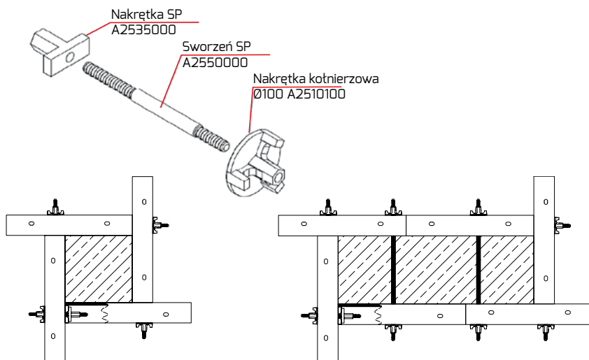
Schemat łączenia płyt
