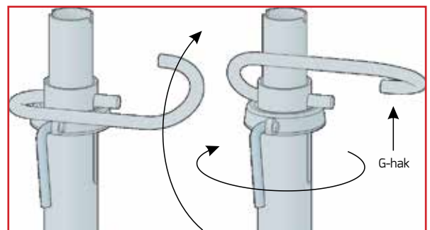
Kolejność postępowania przy odciążaniu podpory przy użyciu G-haka
