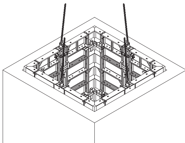
Rys. 7.12 – Demontaż segmentu wewnętrznego
