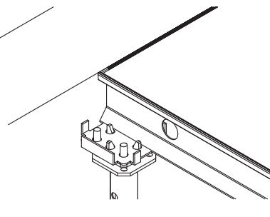
Rys. 14.9 – Podparcie głowicą wsporczą z nakładką głowicy przy ścianie budynku
