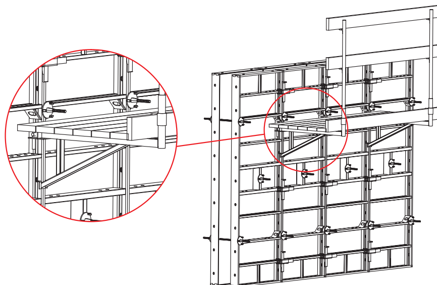
Rys. 3.24 – Fragment zmontowanego pomostu roboczego
